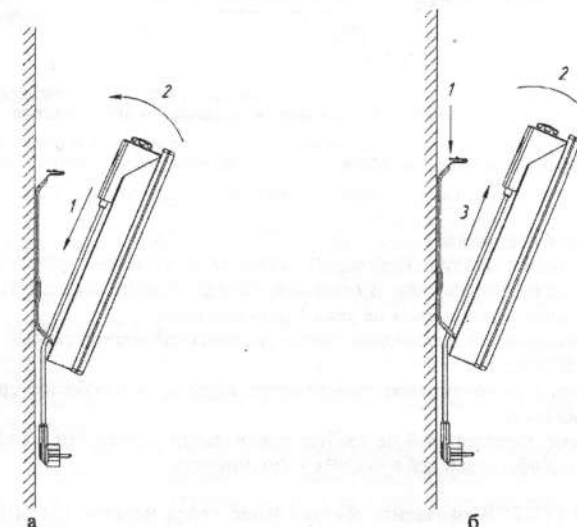
Рисунок 6 – Крепление прибора к кронштейну
