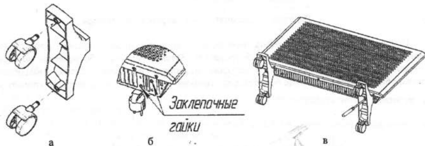
Рисунок 7 - Монтаж ножек напольного обогревателя.
