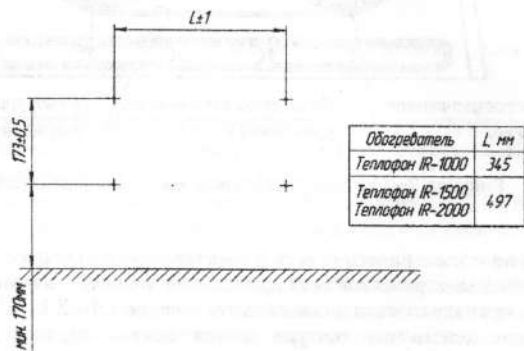
Рисунок 4 - Разметка отверстий для навеса обогревателя.
